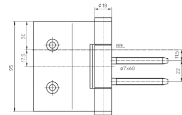
Vorderansicht
